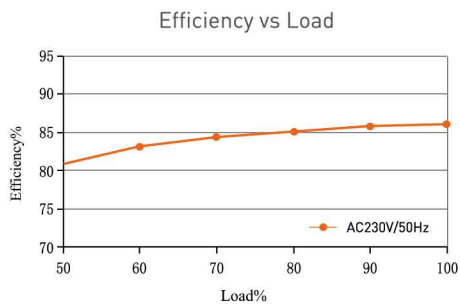
DIM20-12V-200W
