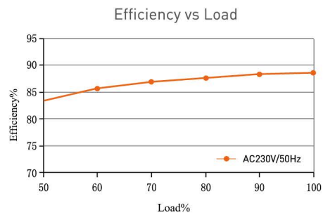
DIM20-24V-200W
